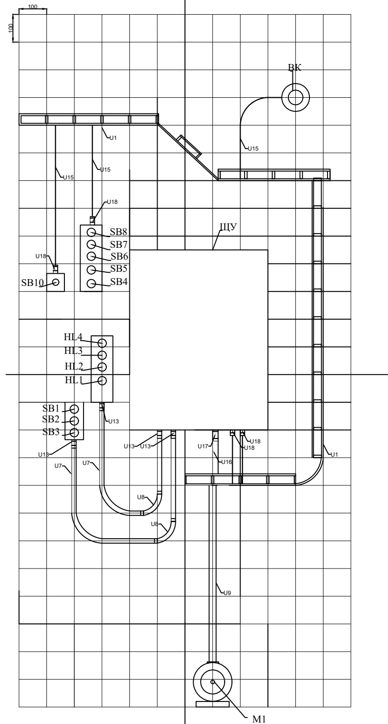
Монтажная схема вид "В"
