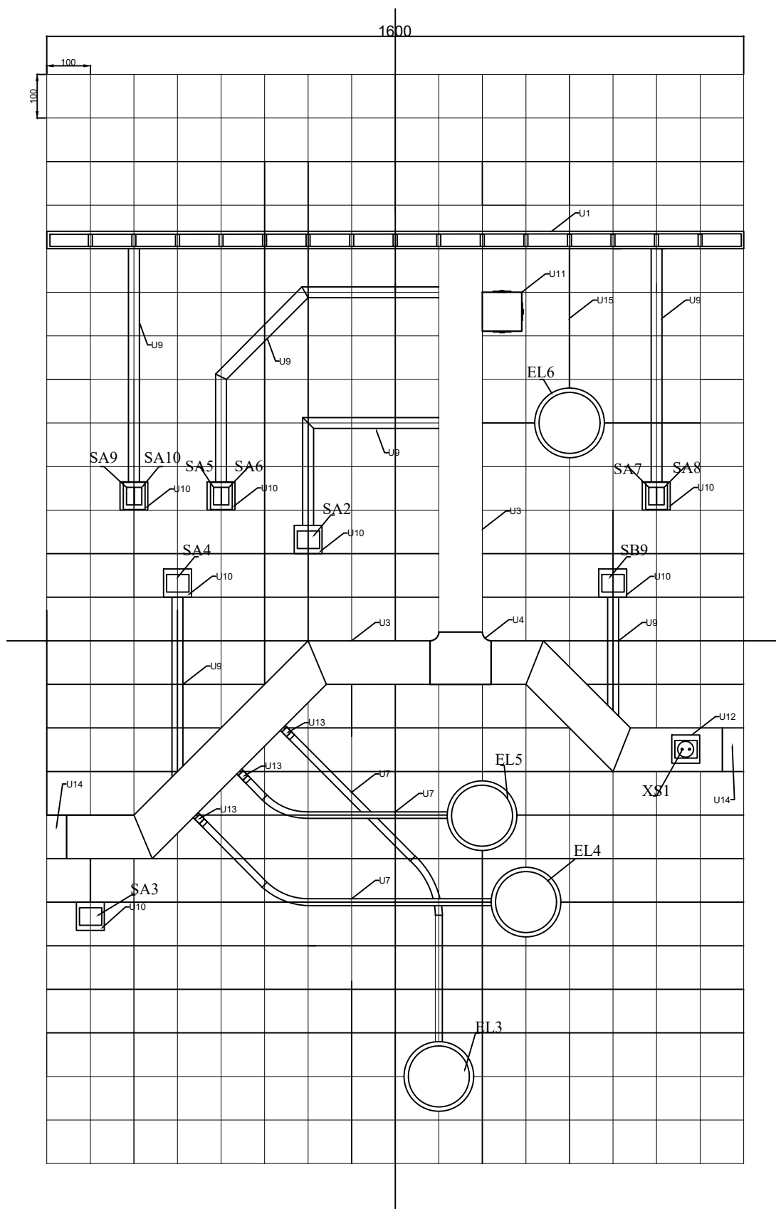
Монтажная схема вид "Б"
